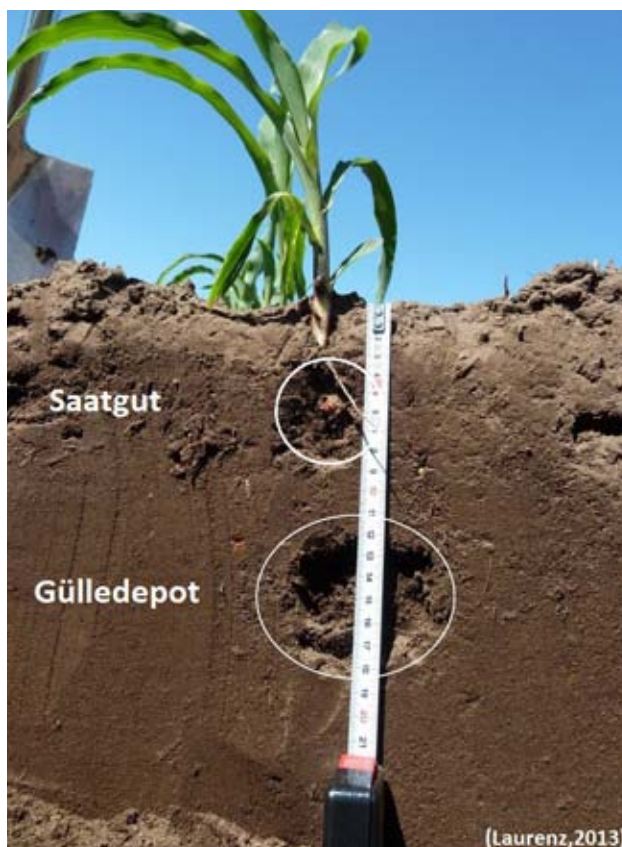
Abb. 2: Lage des Düngerdepots im Boden
